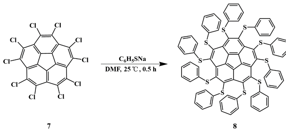
图 6 由十氯碗烯 (7) 制备十苯硫基碗烯 (8)
