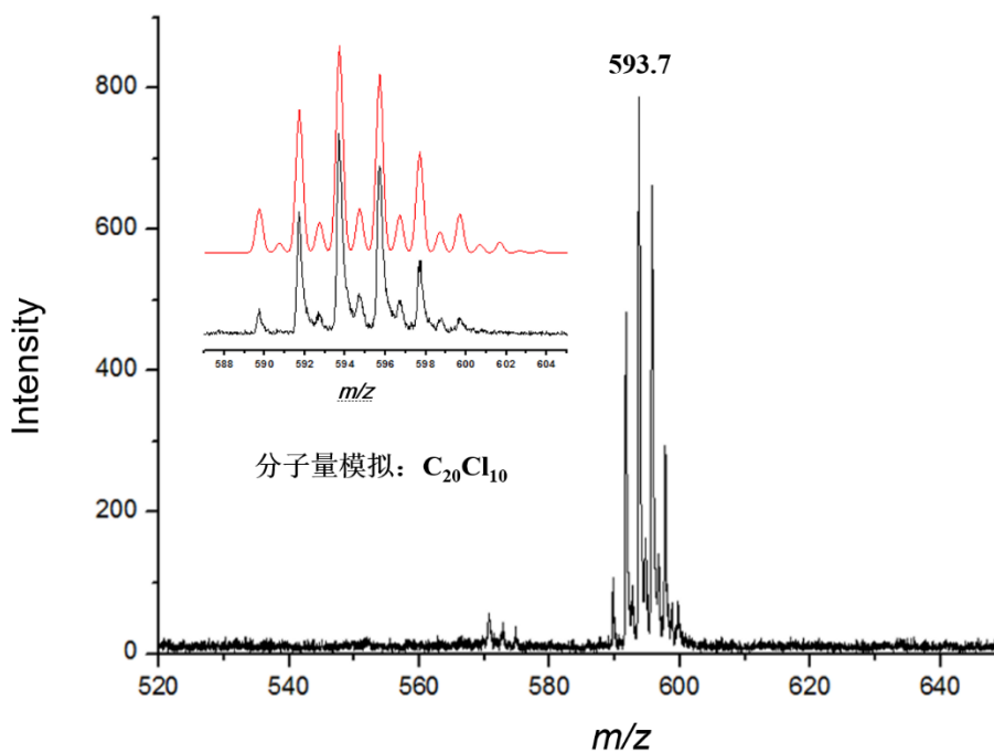
图5 十氯代碗烯 (7) 的 MALDI-TOF-MS 谱图
