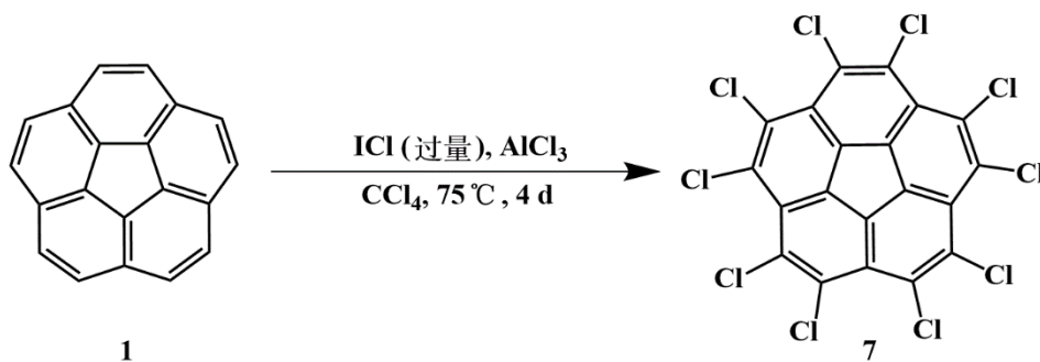
图4 由碗烯 (1) 制备十氯代碗烯 (7) 的新型方法
