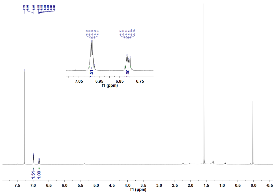
图8 十苯硫基碗烯 (8) 的 ^1\text{H} NMR 谱图
