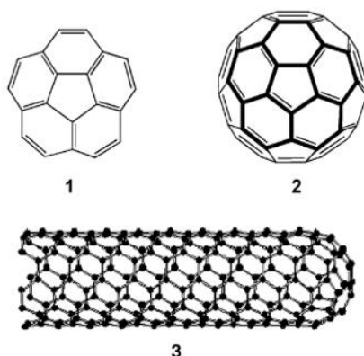
图 1 碗烯 (1)、富勒烯 (2) 和碳纳米管 (3)
