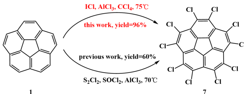
图 3 十氯代碗烯制备方法对比
