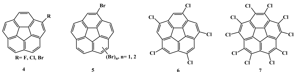
图 2 碗烯的卤代衍生物
