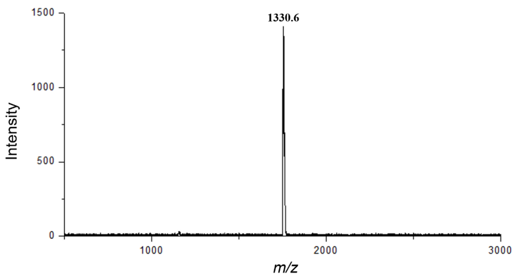
图7 十苯硫基碗烯 (8) 的 MALDI-TOF-MS 谱图
